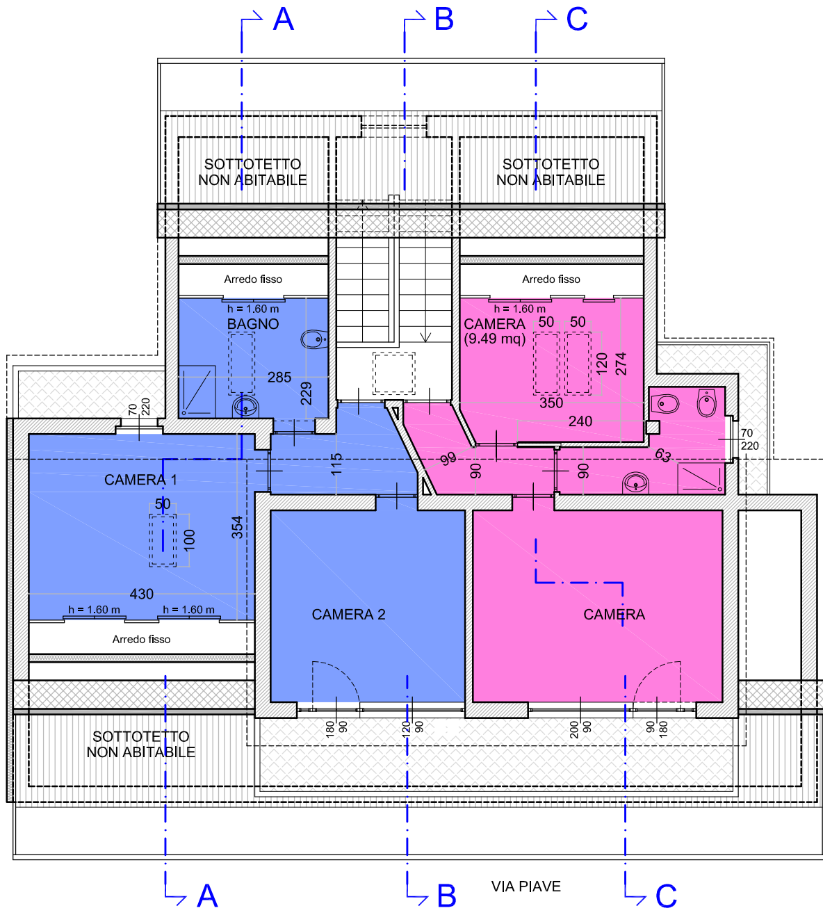
PIANTA PIANO SOTTOTETTO - Scala 1:100 -
