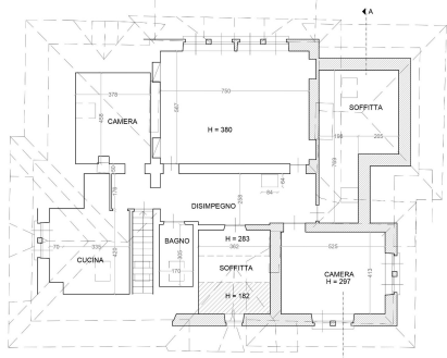
PIANTA PIANO TERZO Scala 1:100
