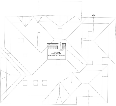
PIANTA TERRAZZA CON ACCESSO DAL PIANO SOTTOTETTO Scala 1:100
