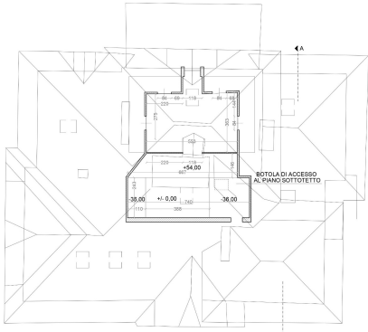
PIANTA PIANO SOTTOTETTO Scala 1:100
