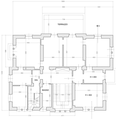
PIANTA PIANO SECONDO Scala 1:100
