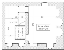
PIANTA PIANO INTERRATO Scala 1:100
