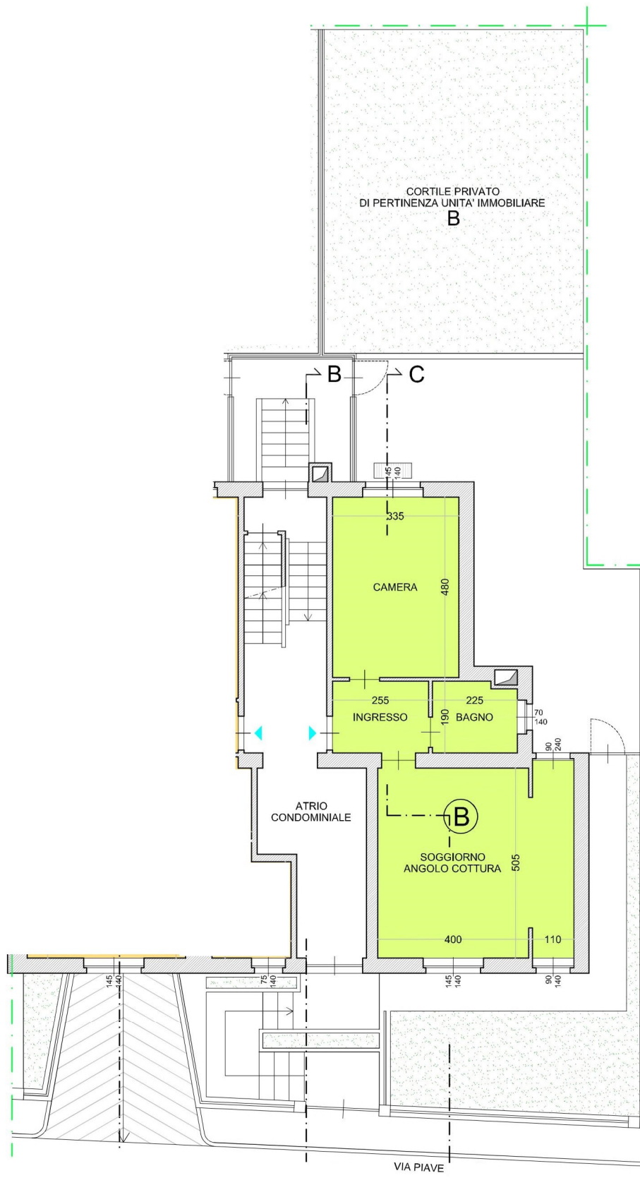
PIANTA PIANO RIALZATO
