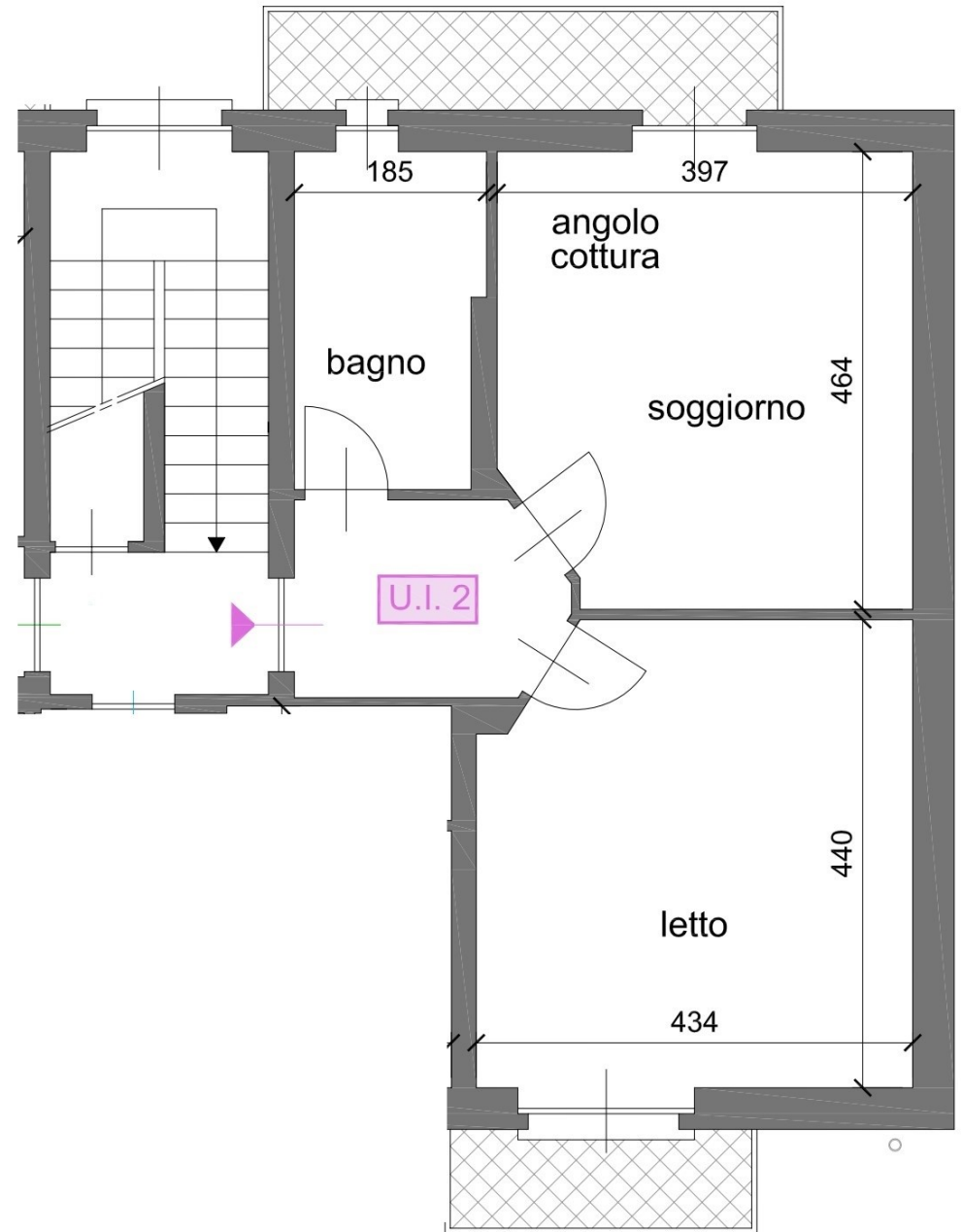
PIANTA PIANO TERZO
