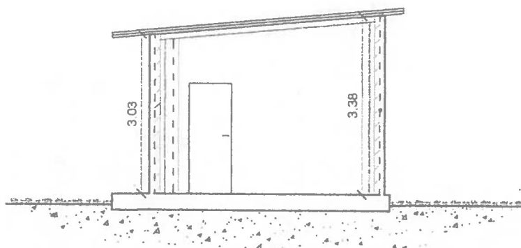
SEZIONE
