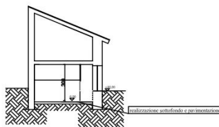
SEZIONE IN PROGETTO Scala 1:100
