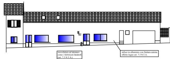
PROSPETTO SU STRADA IN PROGETTO Scala 1:100
